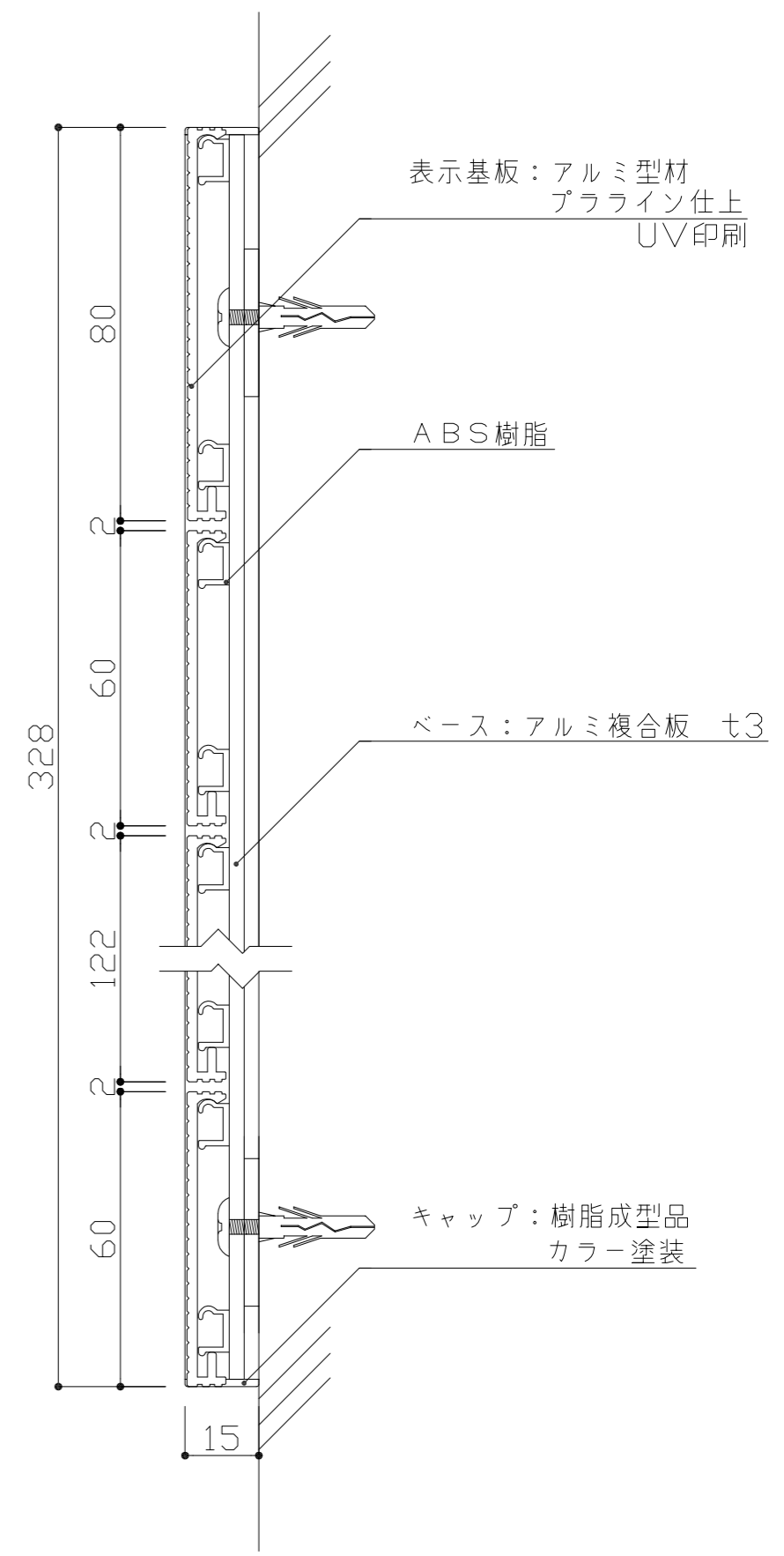
※ 表示基板：プラライン仕上 部分詳細
