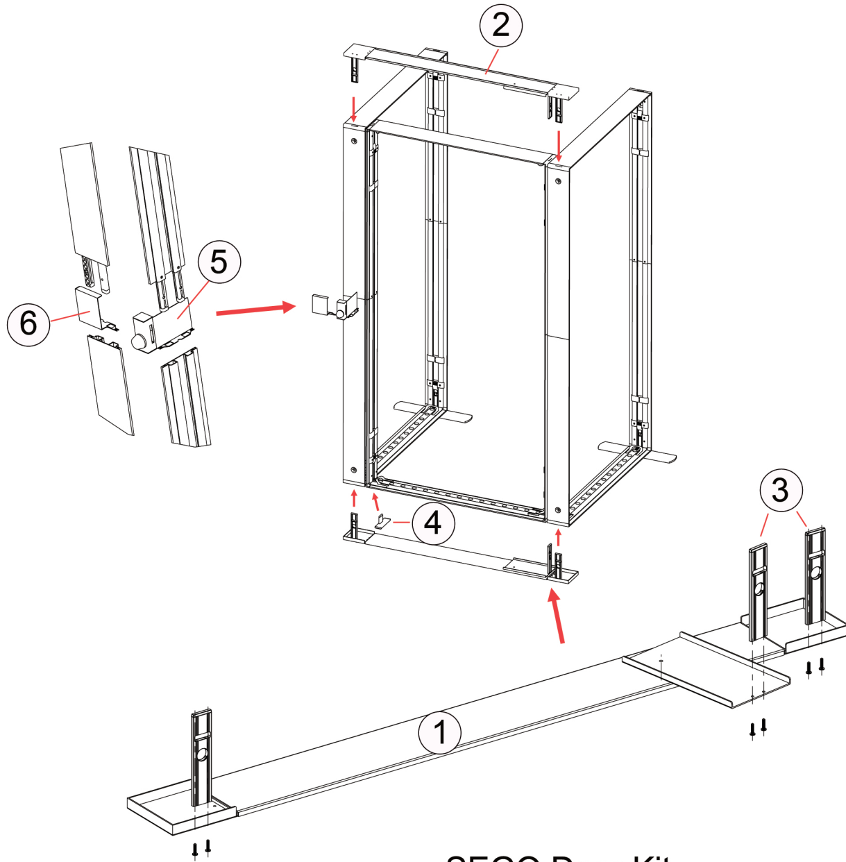
SEGO Door Kit Option 1
